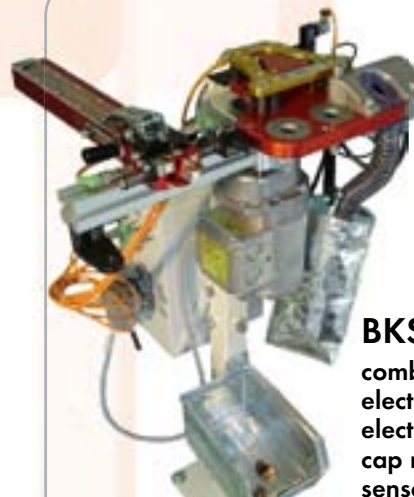
BKS 5810 combi unit - electrode changing system / electrode tip dresser with cap magazine and control sensor (double head) Kombiniertes Kappenwechsel- / Frässystem mit Magazin und Kontrollsensoren (Ausführung Doppelkopf)
